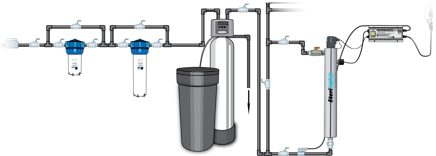
Schéma – installation type au point d'entrée
